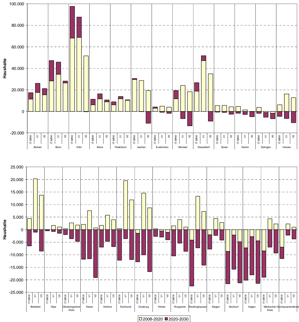
Abbildung 31: Grundlage der Wohnungsnachfrage in den Regionen NRWs bis 2030: Entwicklung der Haushaltszahlen (in den verschiedenen Modellen)
